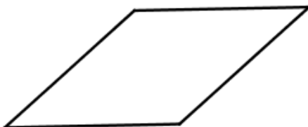
Raute
