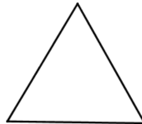
Gleichseitiges Dreieck
