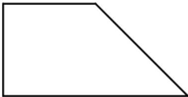
Rechtwinkliges Trapez
