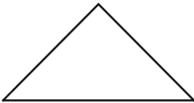
Gleichschenkliges Dreieck
